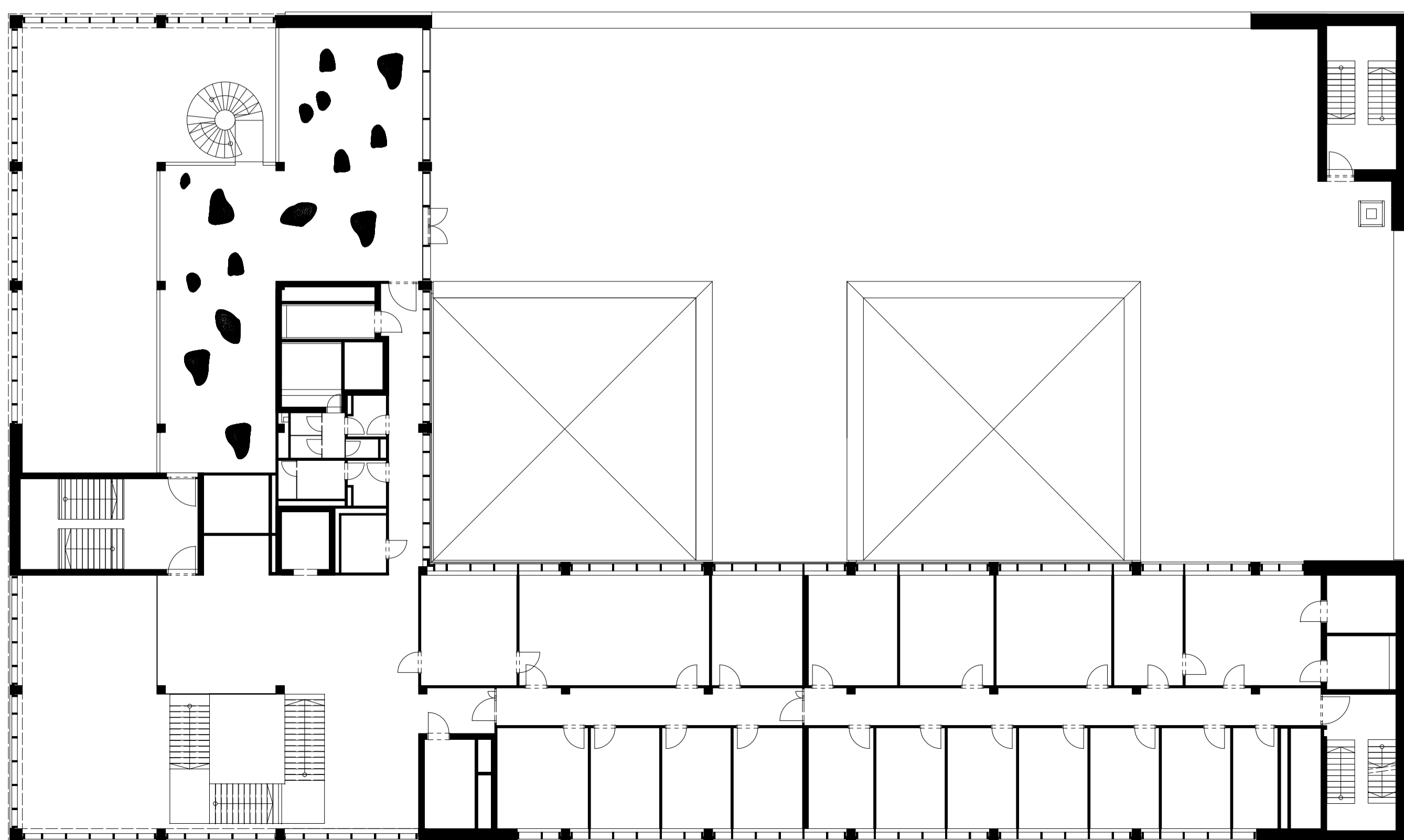
Deckenspiegel_2.Obergeschoss_M 1:200
