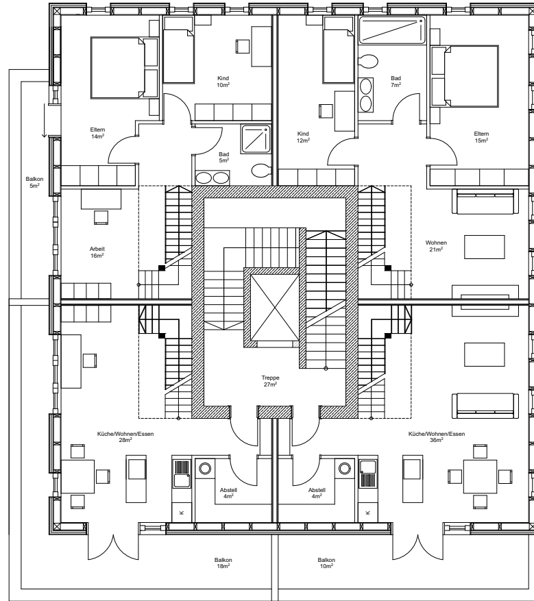
Grundriss_1OG_Wohnturm
