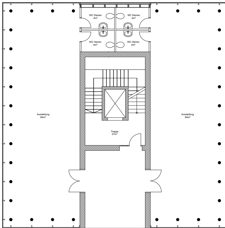
Grundriss_EG_Wohnturm1
