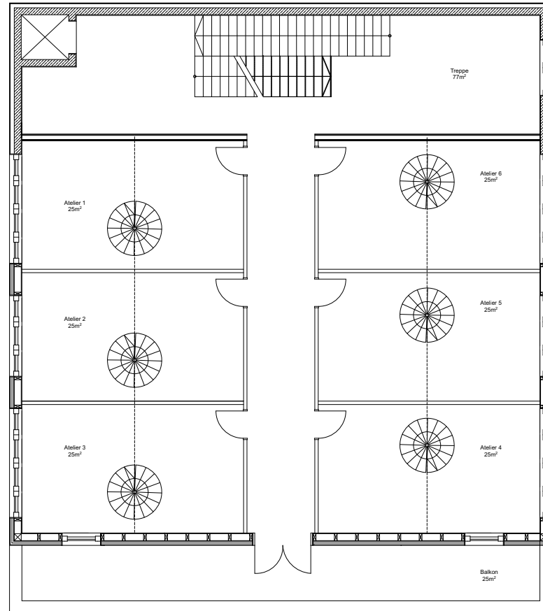
Grundriss_1OG_Künstlerturm
