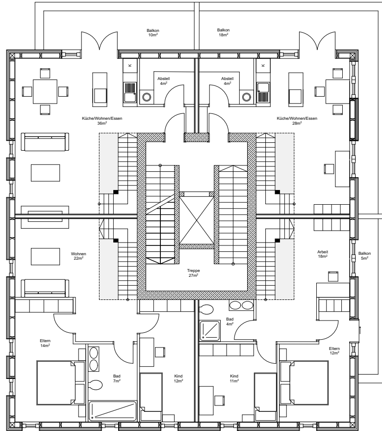
Grundriss_2OG_Wohnturm
