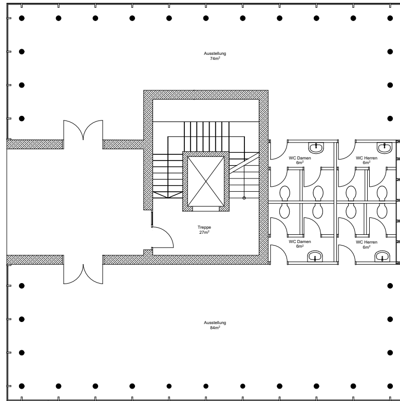
Grundriss_EG_Wohnturm3
