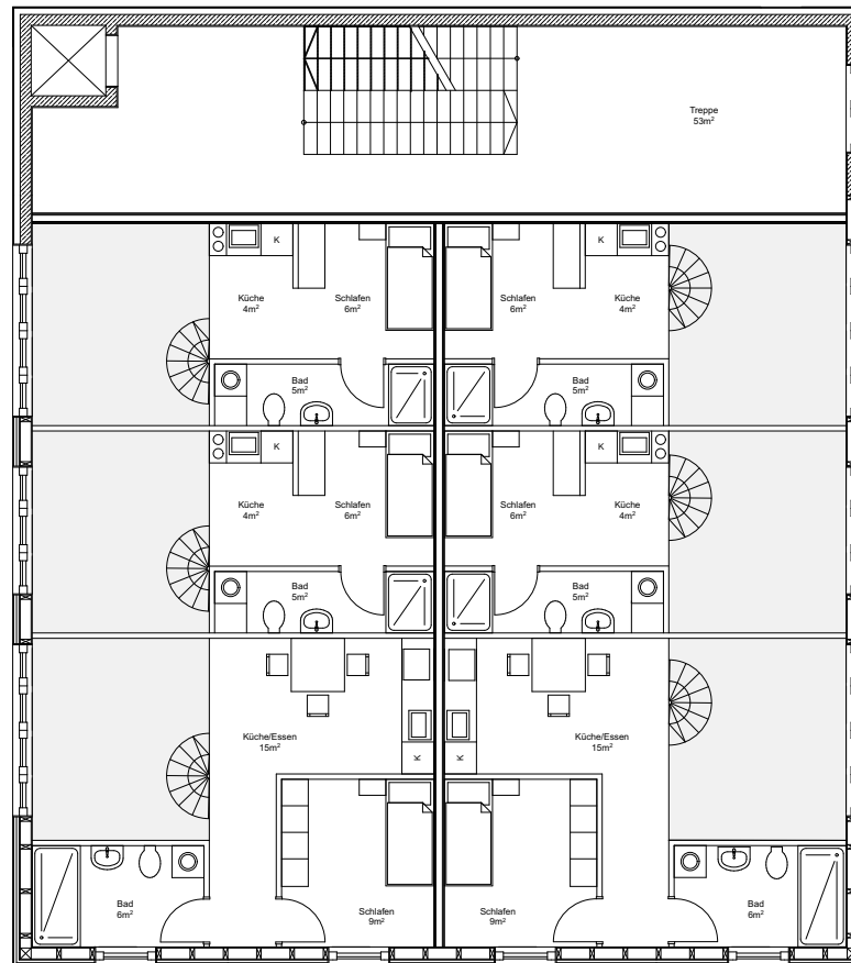
Grundriss_2OG_Künstlerturm
