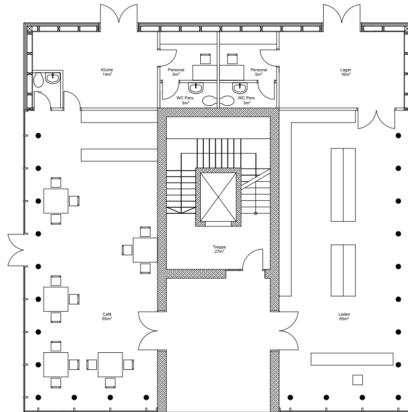
Grundriss_EG_Wohnturm2
