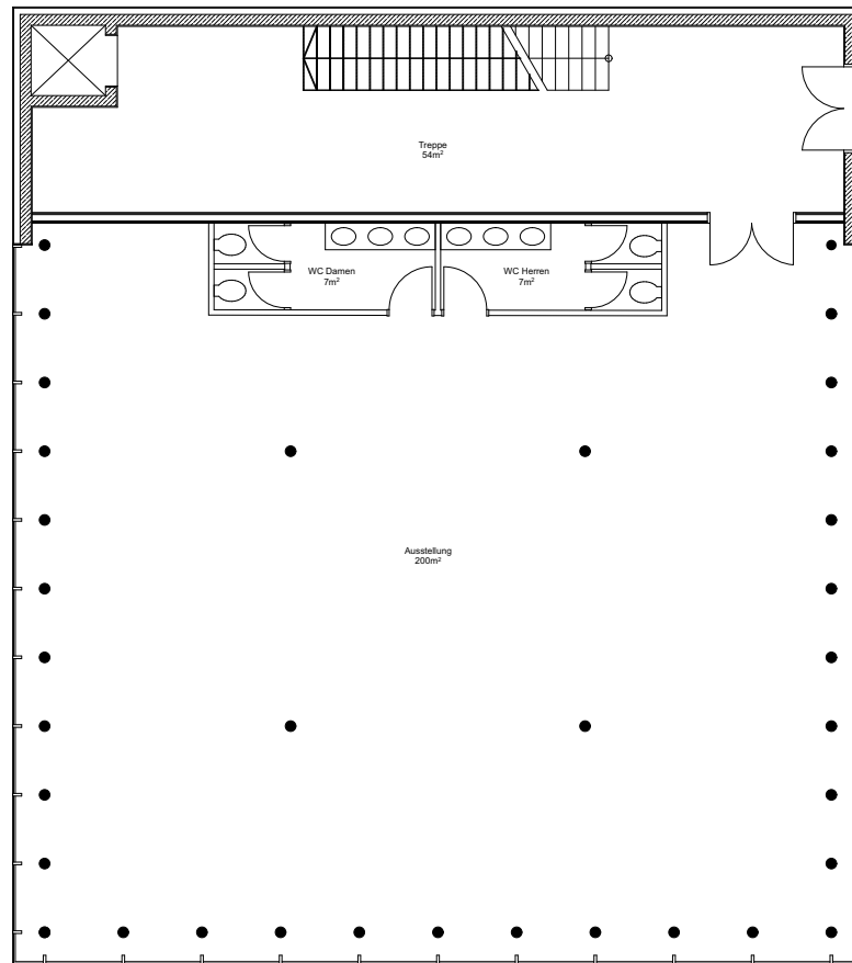
Grundriss_EG_Künstlerturnm
