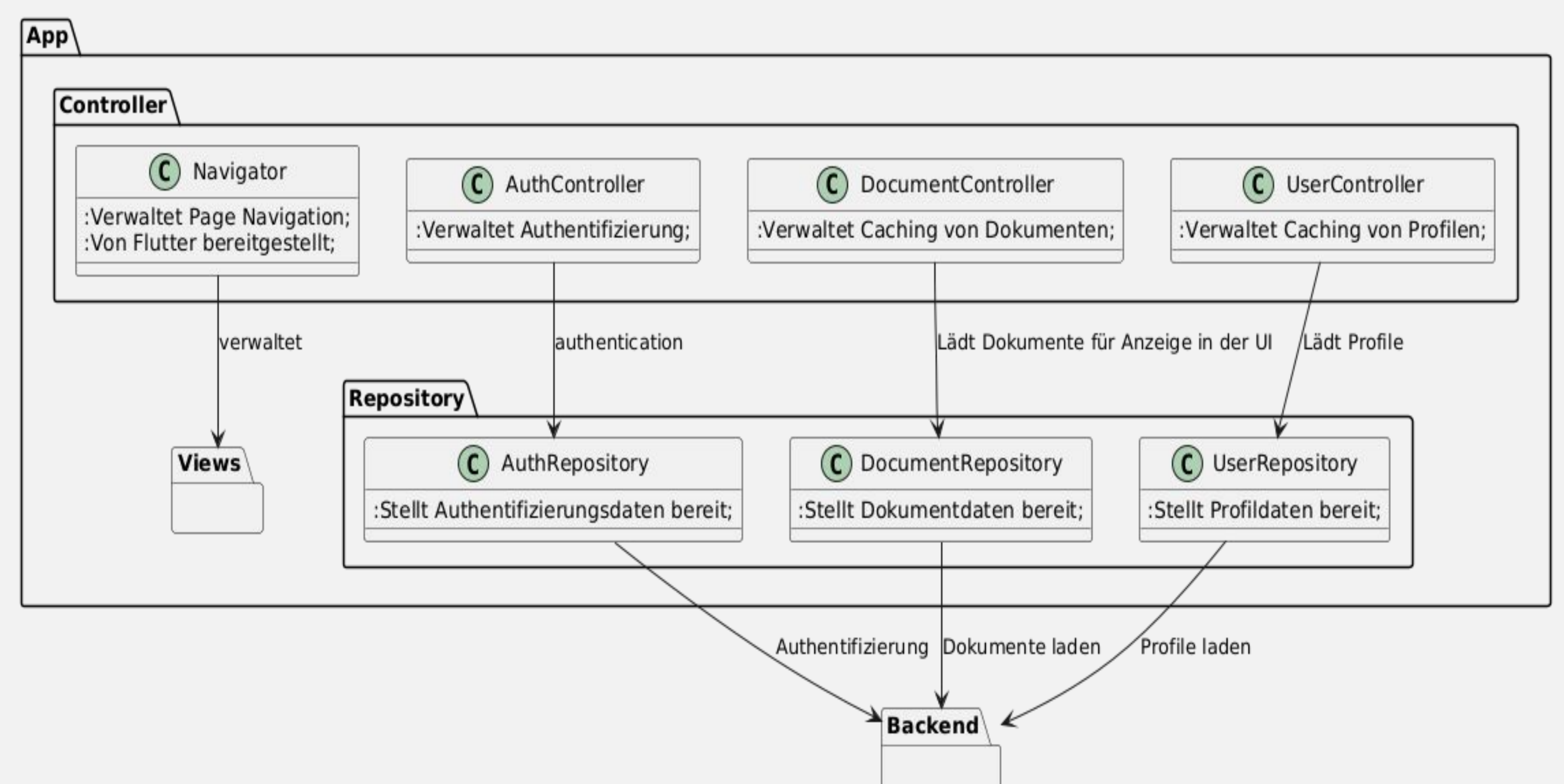
Abb. 5: : Architekturschaubild Frontend
