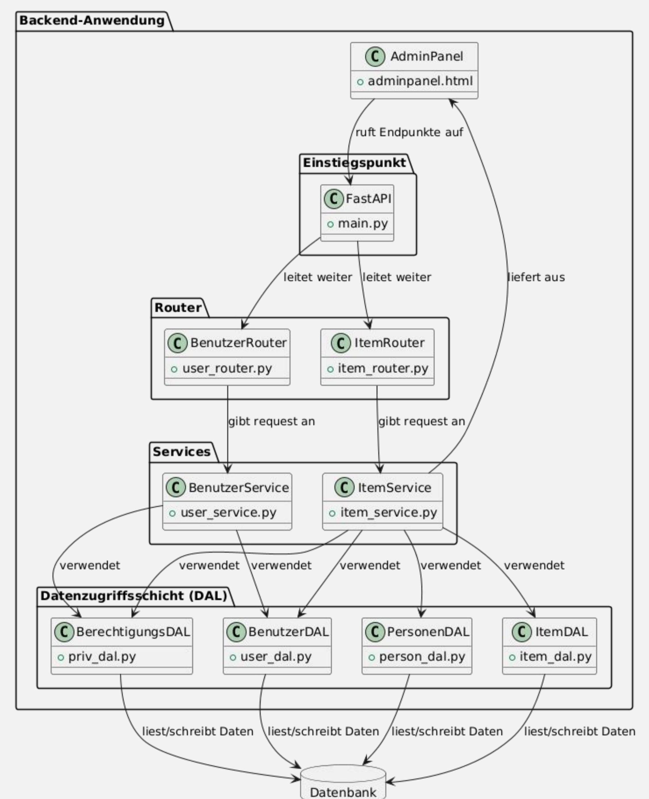
Abb. 4: : Architekturschaubild Backend
